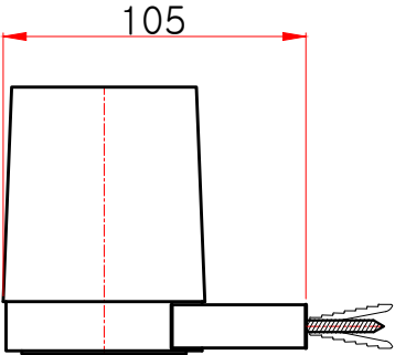
측면도
