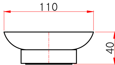
정면도
