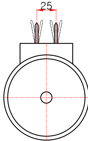
평(윗)면도
