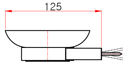
측면도
