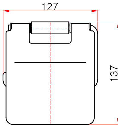
정면도
