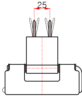
평(윗)면도
