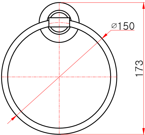
정면도
