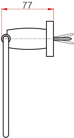
측면도
