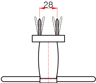
평(윗)면도
