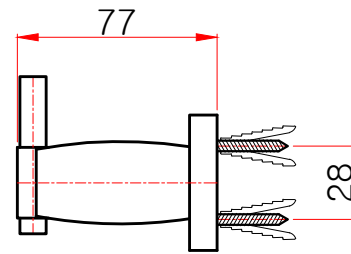
측면도
