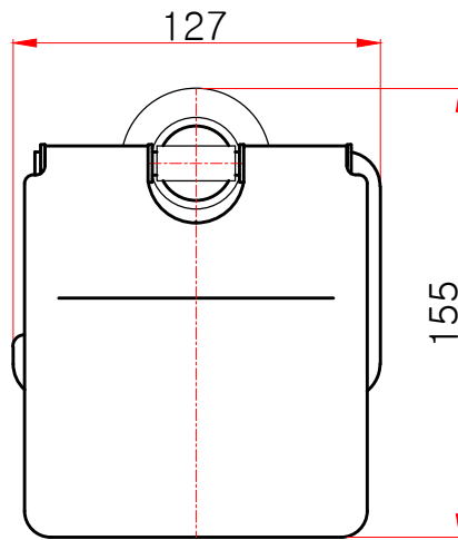
정면도
