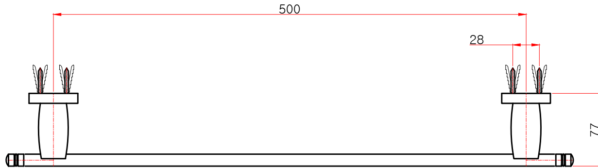
평(윗)면도
