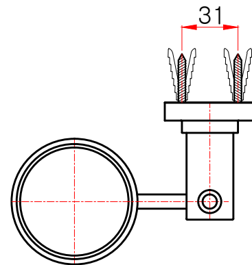
평(윗)면도
