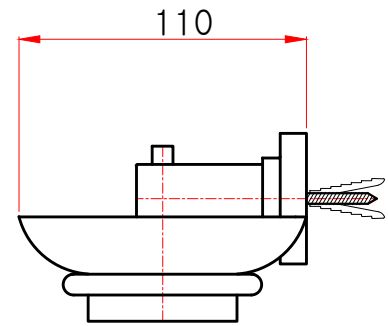
측면도
