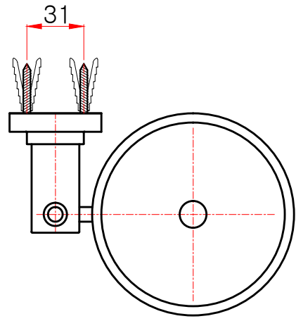
평(위)면도
