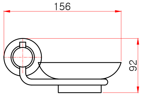
정면도
