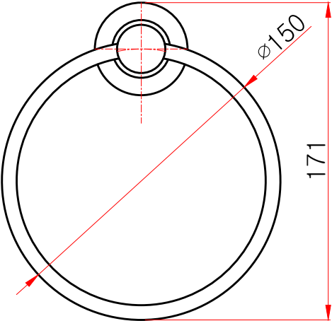
정면도
