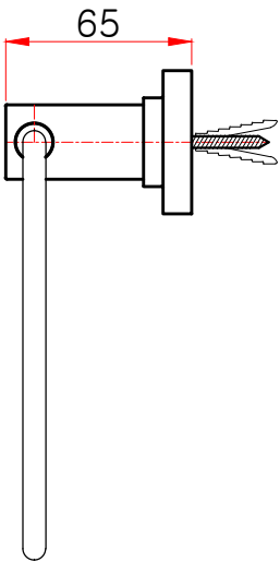
측면도
