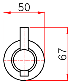
정면도
