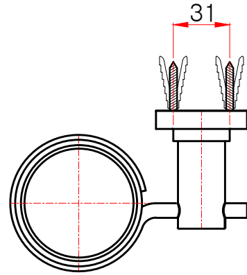
평(윗)면도
