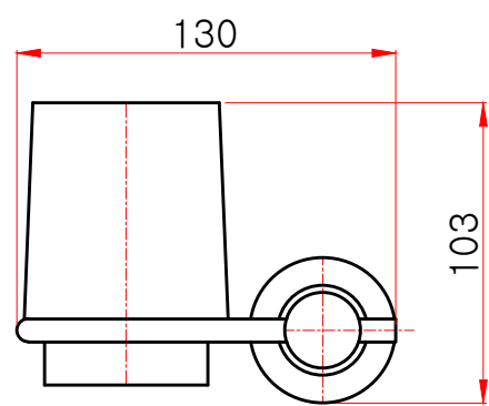
정면도
