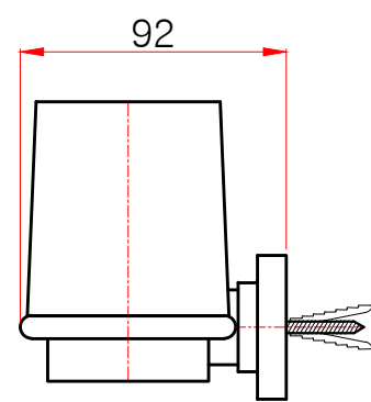
측면도
