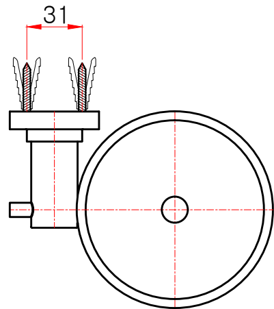
평(윗)면도
