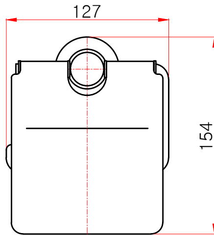
정면도
