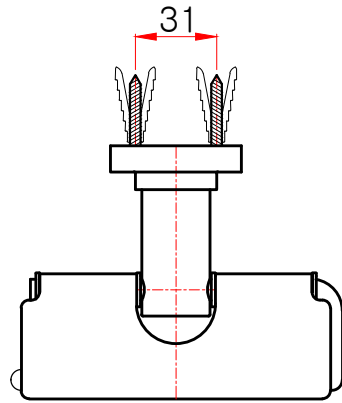
평(윗)면도
