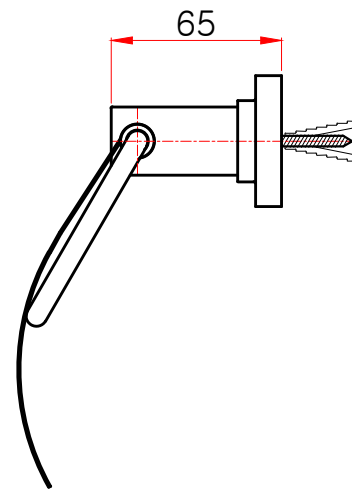
측면도
