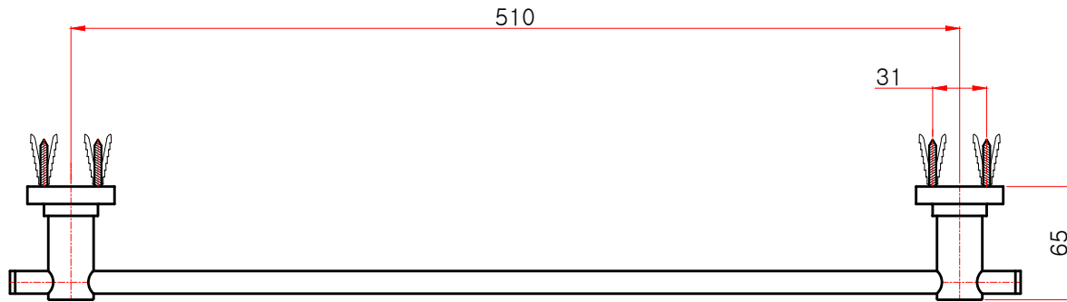
평(윗)면도
