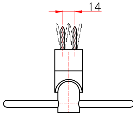
평(윗)면도
