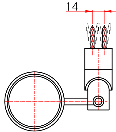
평(윗)면도
