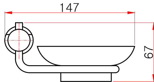
정면도
