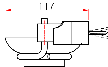
측면도
