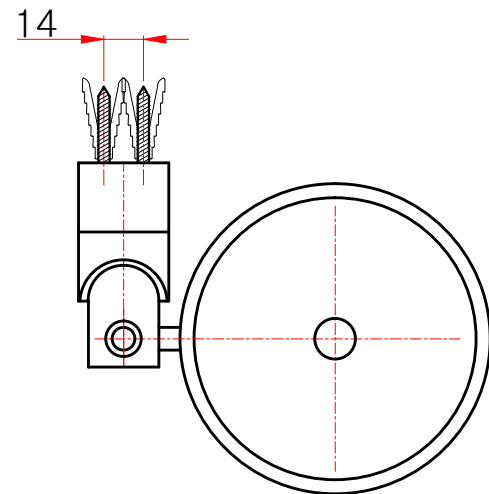
평(윗)면도
