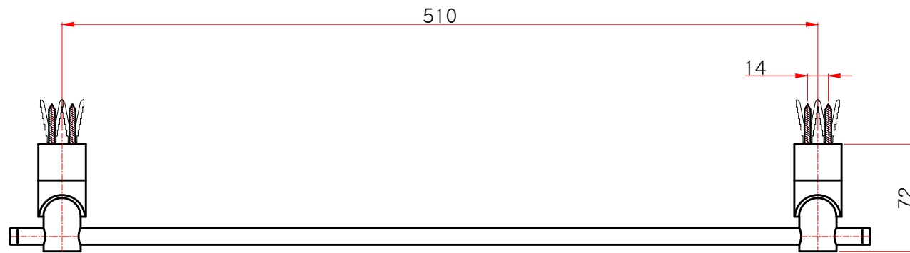
평(위)면도
