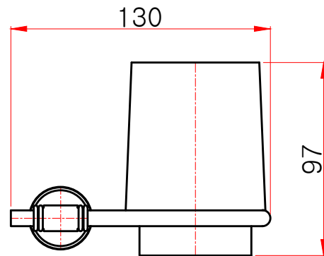
정면도
