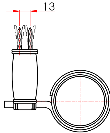
평(윗)면도
