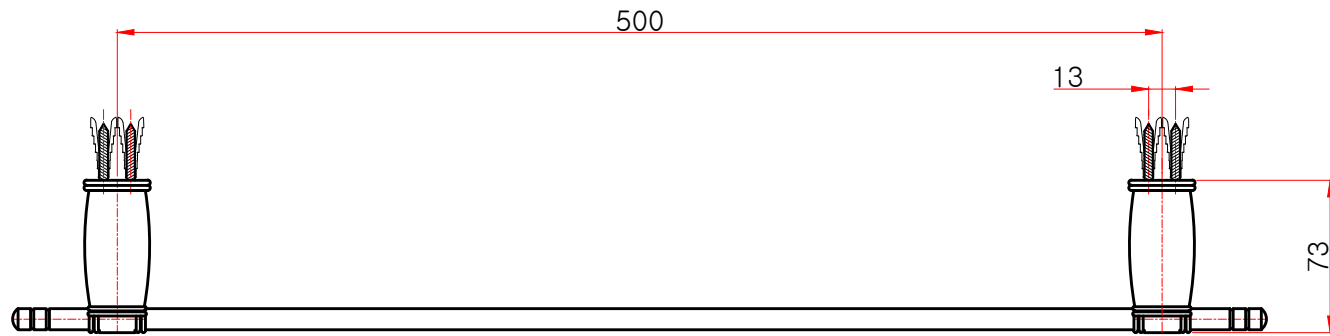
평(윗)면도
