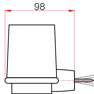
측면도
