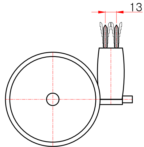
평(윗)면도
