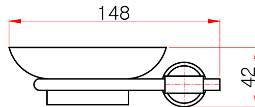
정면도
