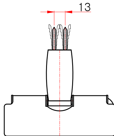
평(윗)면도
