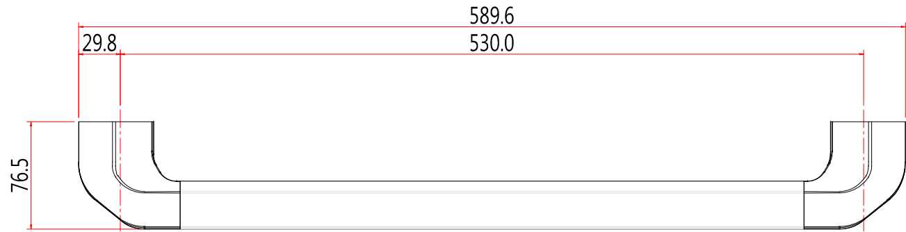
평(윗)면도
