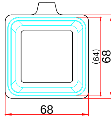
평(윗)면도
