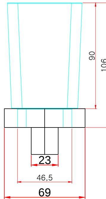
정면도
