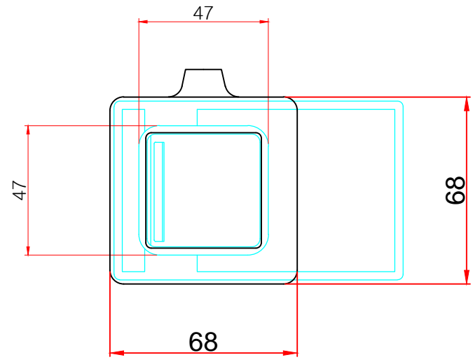
평(윗)면도
