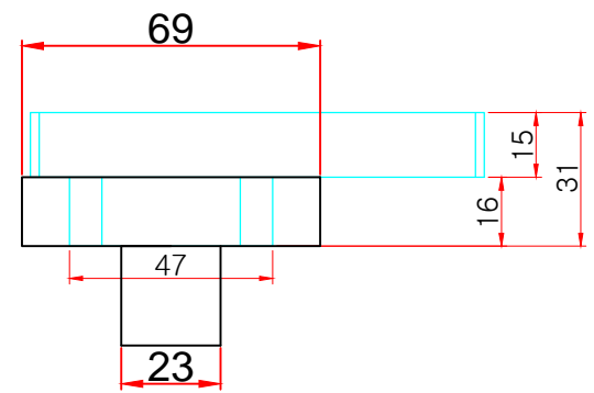
정면도
