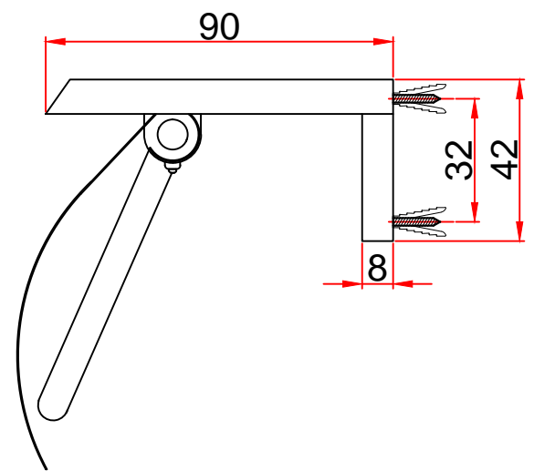
측면도
