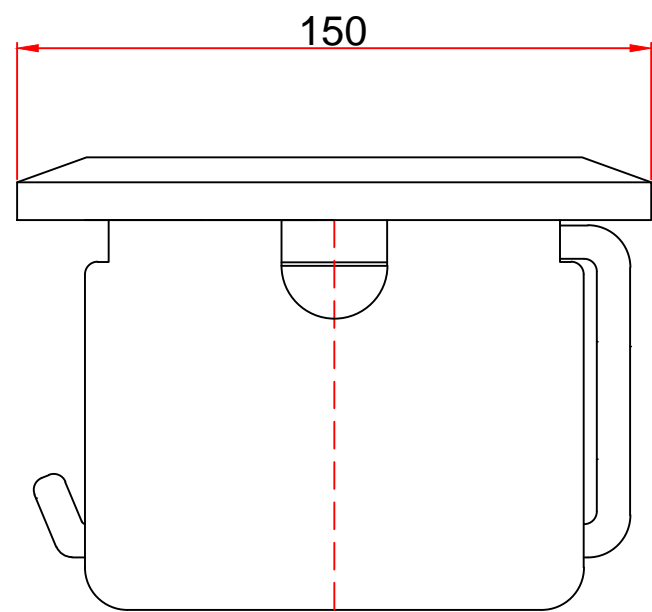
정면도
