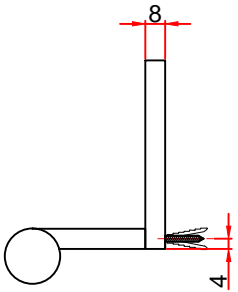
측면도
