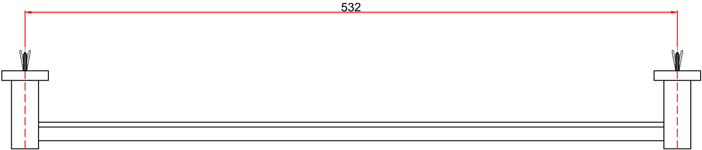
평(위)면도
