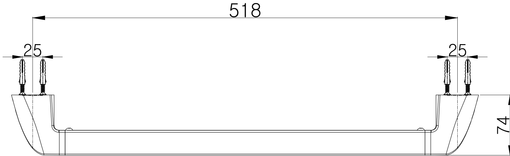
윗면도
