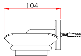
우측면도
