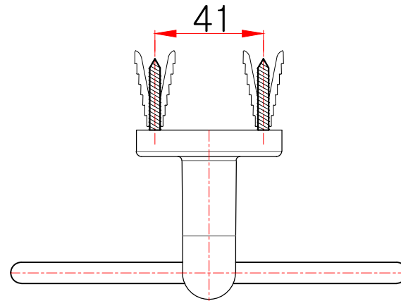
평(윗)면도
