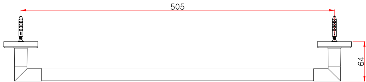
평(횡)면도
