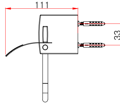
측면도
