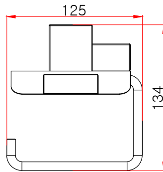
정면도
