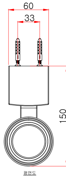
평면도
