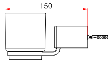
측면도
