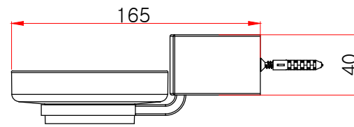
측면도
