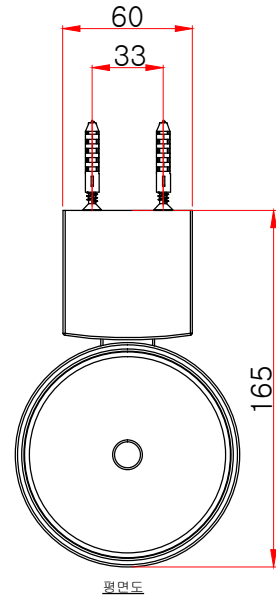
평면도
