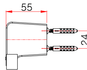
측면도
