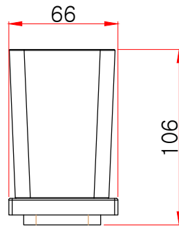
정면도
