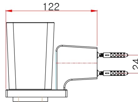
측면도
