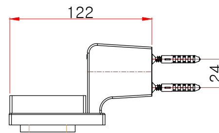
측면도
