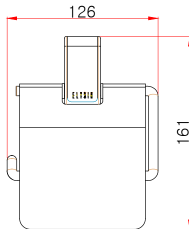
정면도
