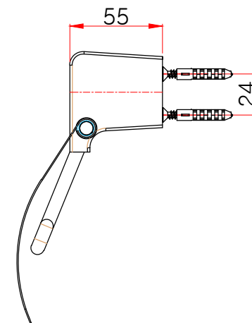
측면도
