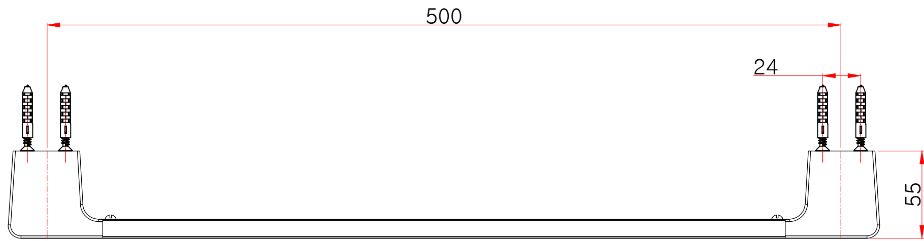
평(윗)면도
