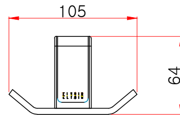
절면도
