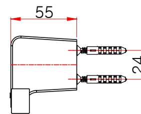
측면도
