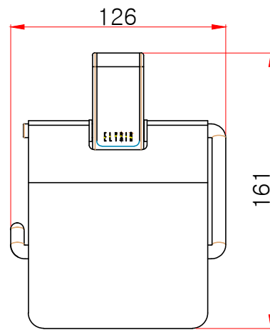
전면도
