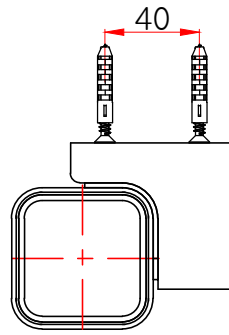
평(위)면도
