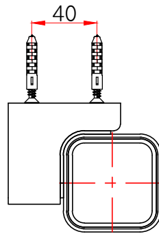
평(위)면도
