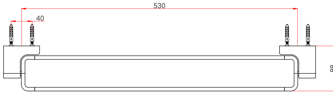
평(위)면도
