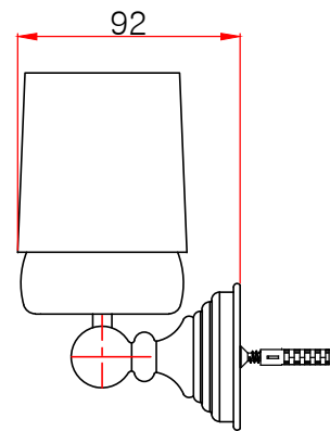
측면도
