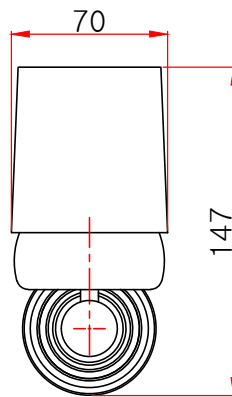
좌면도
