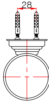
평(윗)면도
