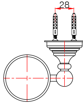
평(윗)면도
