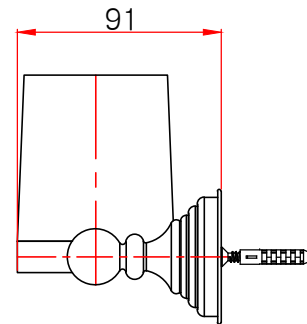
측면도
