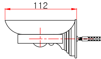
우(右)면도
