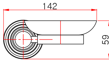
좌(左)면도
