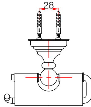
평(위)면도
