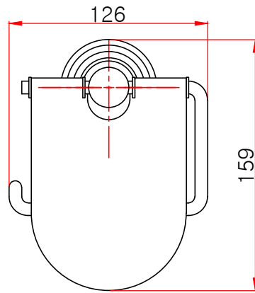
정면도
